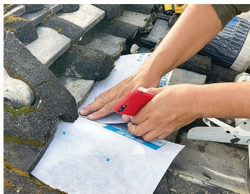
防水シートの挟み込み
