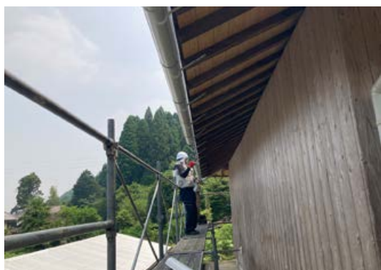
軒樋の取り付け
